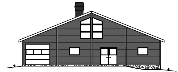
Fasade Vest
